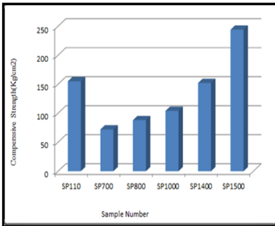
شکل (۱): استحکام فشاری نمونه‌های تف جوشی شده‌ی حاوی سیمان اسپینلی، تحت دماهای ۱۱۰، ۷۰۰، ۸۰۰، ۱۰۰۰، ۱۴۰۰ و ۱۵۰۰ °C.
