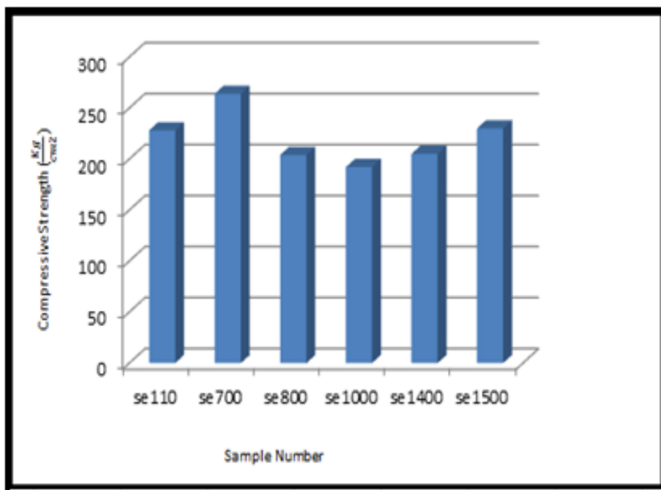
شکل (۱): استحکام فشاری نمونه‌های تف جوشی شده‌ی حاوی سیمان اسپینلی، تحت دماهای ۱۱۰، ۷۰۰، ۸۰۰، ۱۰۰۰، ۱۴۰۰ و ۱۵۰۰ °C.
