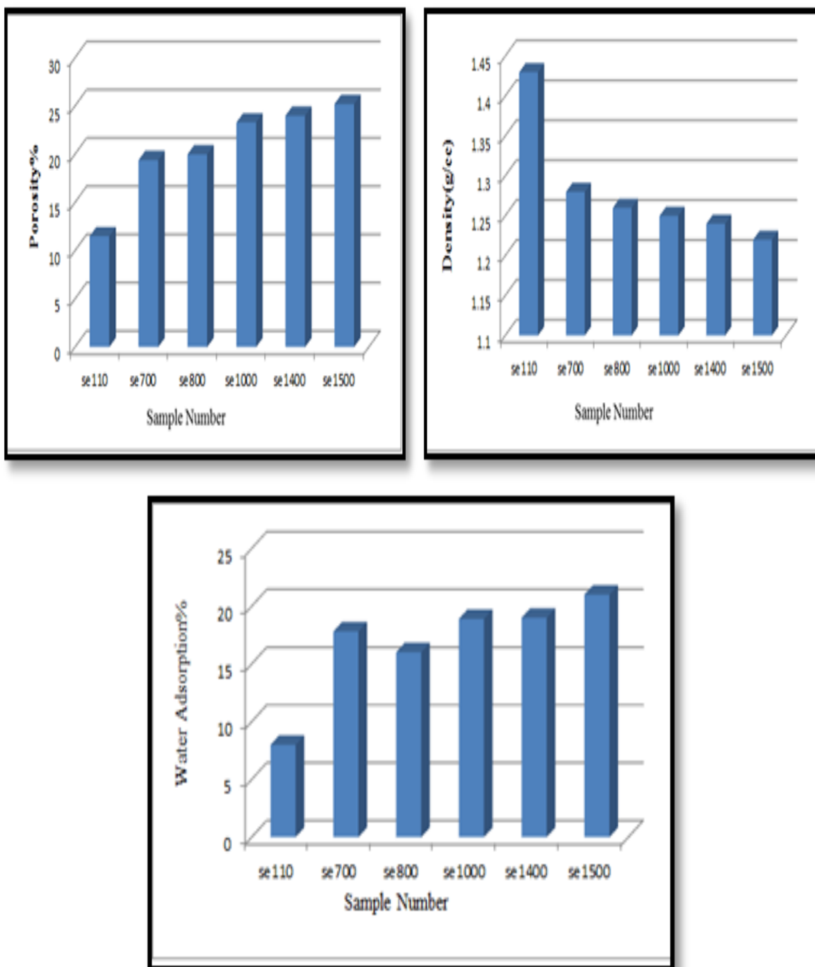
شکل (۴): تاثیر سیمان سکار ۷۱ بر خواص نمونه‌های دیرگدازهای ریختنی در دماهای مختلف
