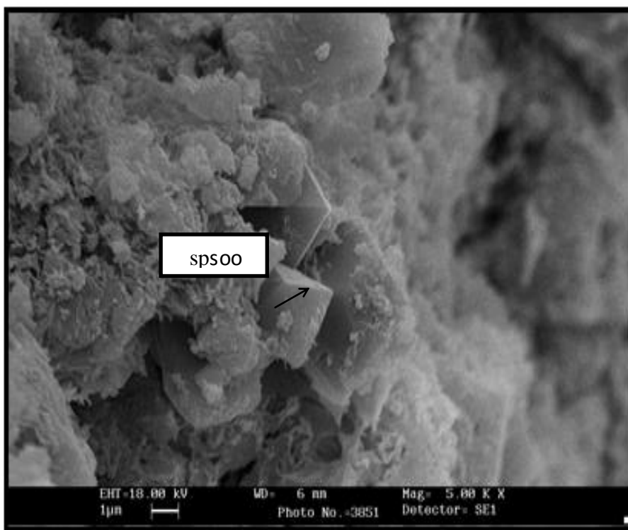
شکل (۱۲): تصویر میکروسکوپ الکترونی از سطح شکست نمونه sp1400 با بزرگنمایی ۵۰۰
