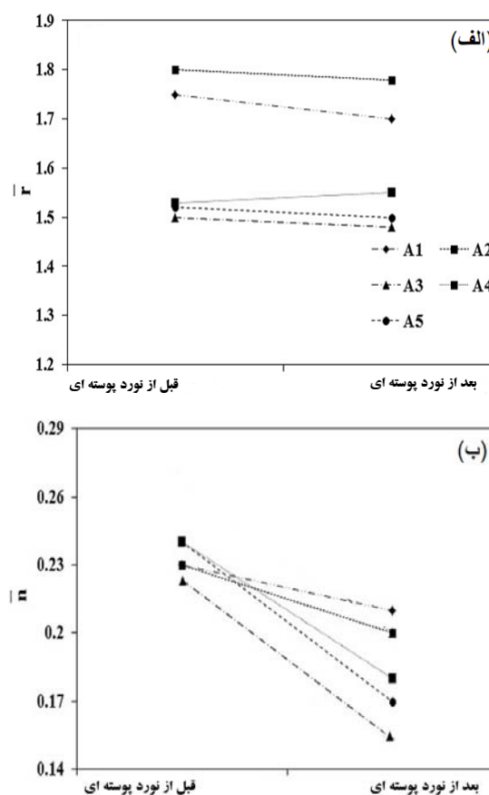
شکل (۳): تغییرات (الف) \bar{\Gamma} و (ب) \bar{n} برای مجموعه (A) قبل و بعد از نورد پوسته‌ای
