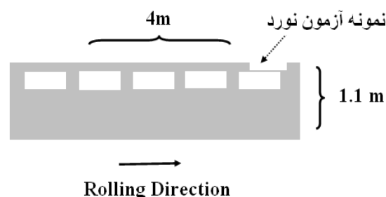
شکل (۲): نحوه آماده سازی ۵ نمونه نورد سری B
