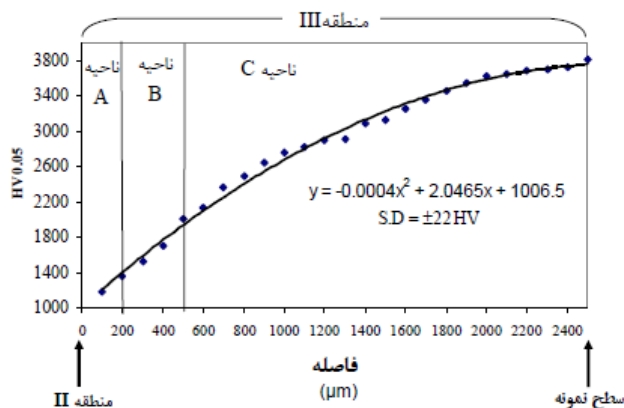
شکل (۸): سختی کاربیدهای اولیه (Cr,Fe)_7C_3 در ۳ ناحیه منطقه III.
