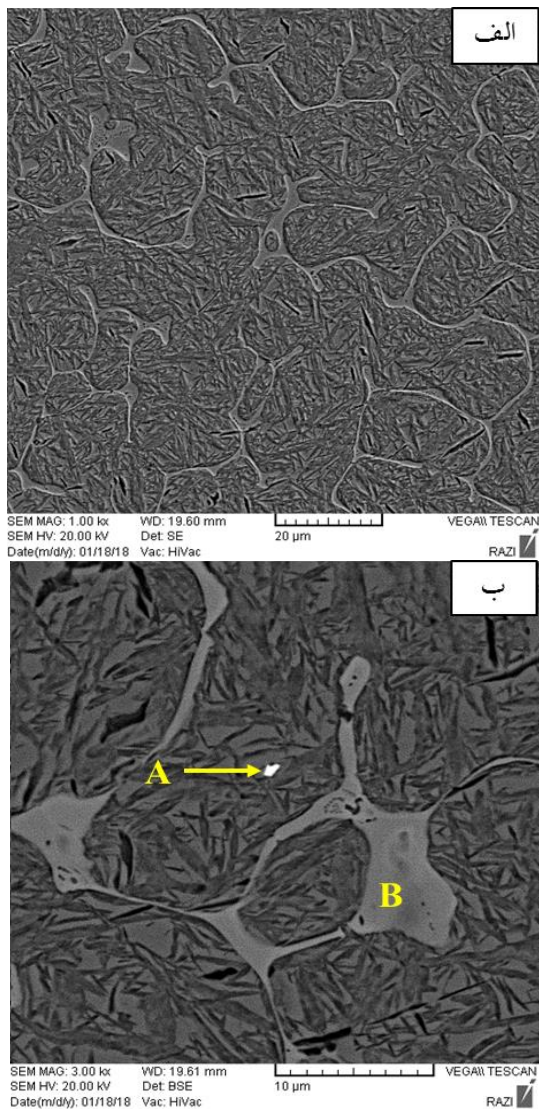
شکل (۲): ریزساختار میکروسکوپ الکترونی نمونه ۱ در دو بزرگنمایی مختلف
