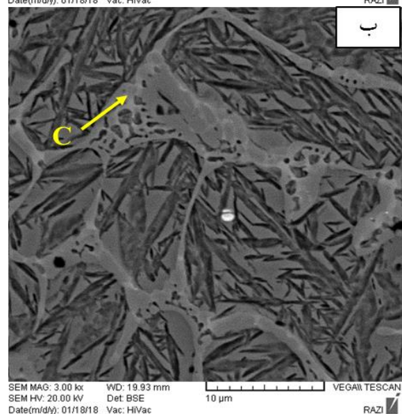
شکل (۳): ریزساختار میکروسکوپ الکترونی نمونه ۲ در دو بزرگنمایی مختلف
