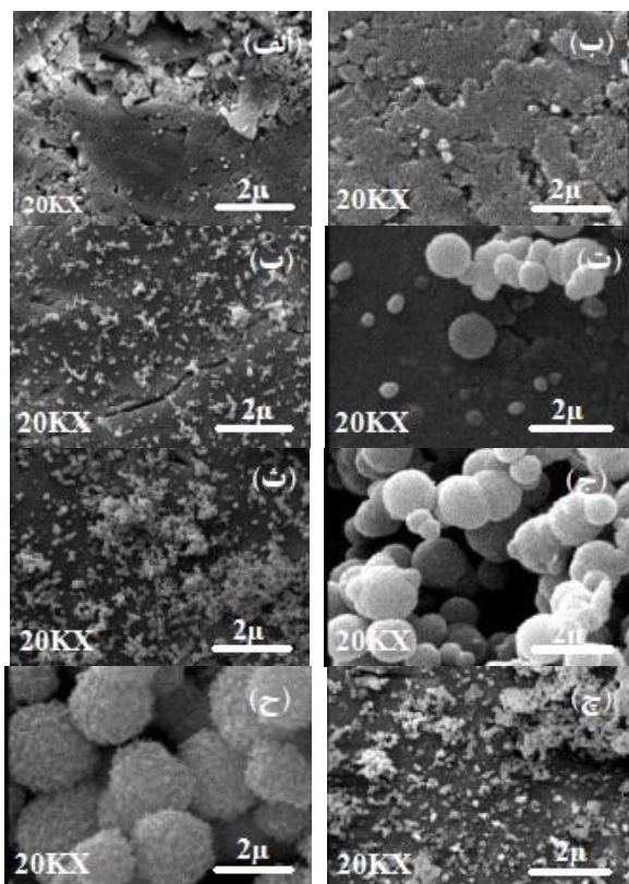
شکل (۸): ریزساختار لایه هیدروکسی آپاتایت ایجاد شده روی سطح S_0 (الف و ب) قبل از غوطه‌وری، پ و ت) پس از ۱ روز غوطه‌وری، ج و ح) پس از ۷ روز غوطه‌وری و چ و ج) پس از ۳۰ روز غوطه‌وری در محلول شبیه‌سازی شده با محیط بدن.
