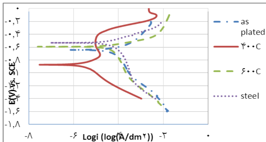
شکل (۱۱): منحنی پلاریزاسیون زیرلایه فولادی و پوشش‌های آلیاژی Co-W حاصل از آبکاری الکتریکی قبل و بعد از عملیات حرارتی
