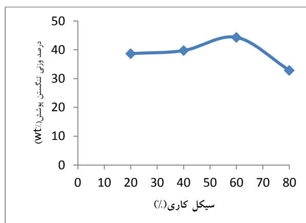
شکل (۶): نتایج آنالیز عنصری پوشش بدست آمده بر حسب سیکل کاری
