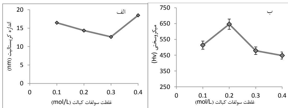
شکل (۴): (الف): نمودار اندازه کریستالیت و (ب): میکروسختی، پوشش‌های بدست آمده بر حسب غلظت سولفات کبالت
