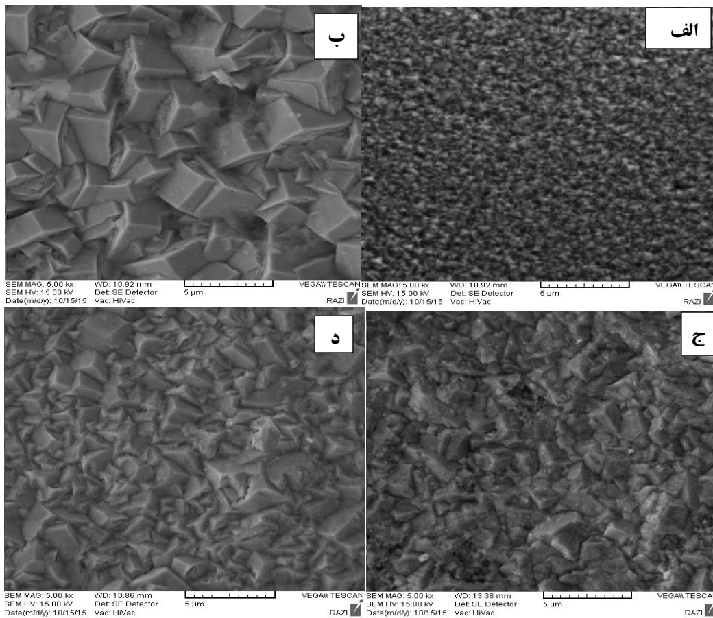
شکل (۱): تصاویر SEM سطح پوشش‌ها در چگالی جریان متوسط 1 \text{ A/dm}^2 ، سیکل کاری ۲۰٪، فرکانس 200 \text{ Hz} و غلظت سولفات کبالت: (الف): ۰/۱، (ب): ۰/۲، (ج): ۰/۳ و (د): 0.4 \text{ mol/l}
