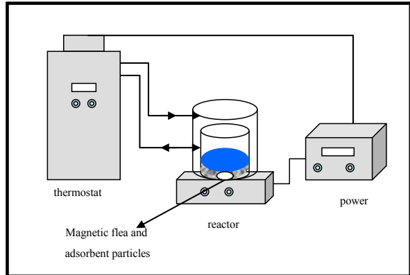
شکل ۲ تصویر شماتیک آزمایش
