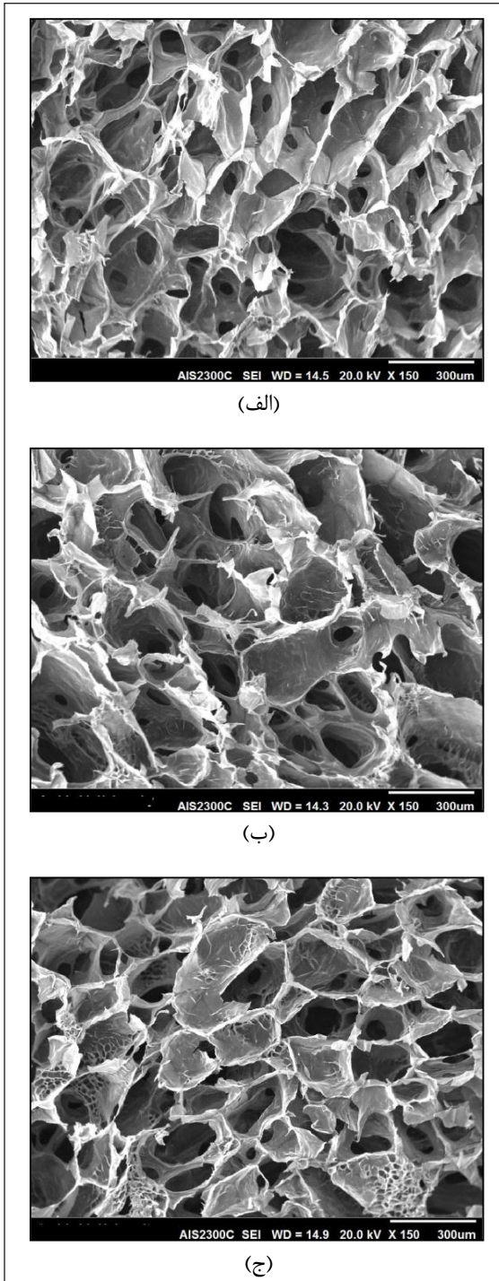
شکل ۵ تصویرهای SEM از داربست‌های کامپوزیتی تهیه شده با نسبت ویسکر کلسیم فسفات به کیتوسان، (الف) ۵:۱ (ب) ۳:۱ (ج) ۱:۱
