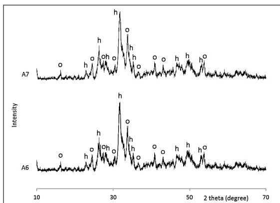
شکل ۲ الگوهای پراش پرتو ایکس نمونه‌های A6 و A7 O، اکتاکلسیم فسفات (Ca_8(HPO_4)_2(PO_4)_4 \cdot 5H_2O) ؛ h، هیدروکسی آپاتیت (Ca_{10}(PO_4)_6(OH)_2) و اکتاکلسیم فسفات
