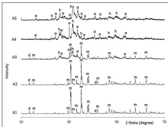
شکل ۱ الگوهای پراش پرتو ایکس نمونه‌ها، A1 تا A5 d، براشیت (CaHPO_4 \cdot 2H_2O) ; m، موتنیت (CaHPO_4) ; O، اکتاکلسیم فسفات (Ca_8(HPO_4)_2(PO_4)_4 \cdot 5H_2O) ؛ h، هیدروکسی آپاتیت (Ca_{10}(PO_4)_6(OH)_2) و اکتاکلسیم فسفات
