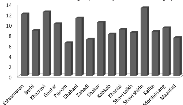
شکل ۸ مقایسه بازده روغن هسته خرما با شرایط بهینه استخراج (واریتہ زاهدی، S/L=3/1 ، حلال پترولیوم اتر، ۱،۵ ساعت بازروانی و ۱،۵ ساعت سوکسله با آسیاب دوباره پودر هسته و اندازه دانه‌های هسته ۱ mm)
