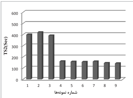
شکل ۴ تغییرات زمان برشته‌گی آمیزه‌ها با افزایش مقدار دوده بازیافتی
