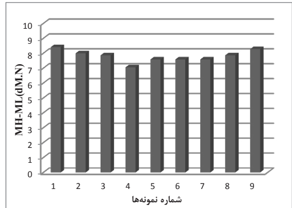
شکل ۲ تغییرات چگالی پیوندهای عرضی آمیزه‌ها با افزایش مقدار دوده بازیافتی
