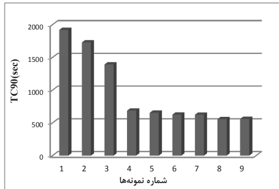
شکل ۳ تغییرات زمان بهینه پخت آمیزه‌ها با افزایش مقدار دوده بازیافتی
