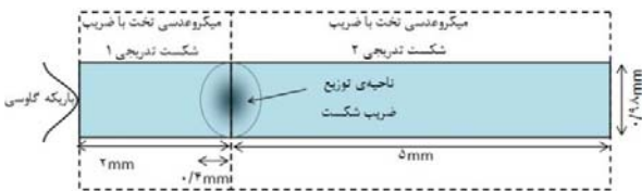
شکل ۳. مشخصات ابعادی و نحوه‌ی قرارگیری دو میکروعدسی با ضریب شکست تدریجی جفت شده.
