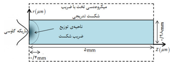
شکل ۱. مشخصات ابعاد میکروعدسی تخت با ضریب شکست تدریجی
