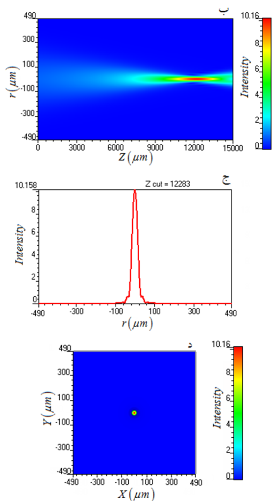
شکل ۵. الف. توزیع شدت پرتوی گاوسی ورودی به میکروعدسی تخت با ضریب شکست تدریجی در سطح مقطع XY . ب. توزیع دو بعدی شدت پرتوی گاوسی در تمام ناحیه ی شبیه سازی شده، ج. شدت یک بعدی پرتوی گاوسی شبیه سازی شده در نقطه کانونی، د. توزیع شدت پرتوی گاوسی کانونی شده با میکروعدسی تخت با ضریب شکست تدریجی در سطح مقطع XY
