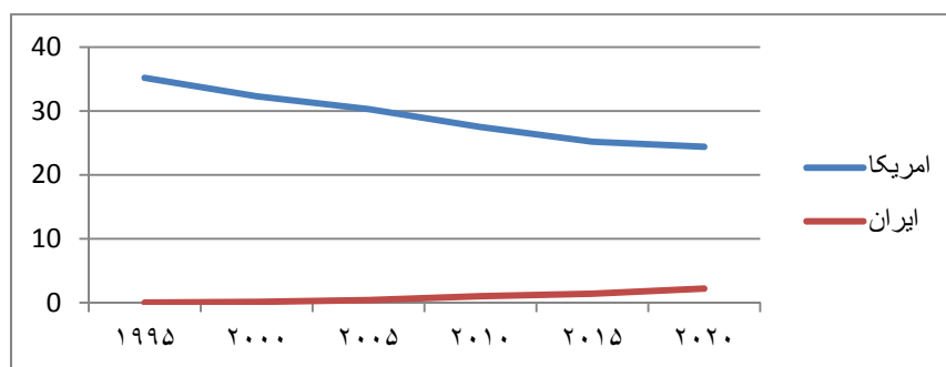
نمودار ۱. سهم تولیدات ایران و آمریکا از کل تولیدات جهان در پایگاه web of science
