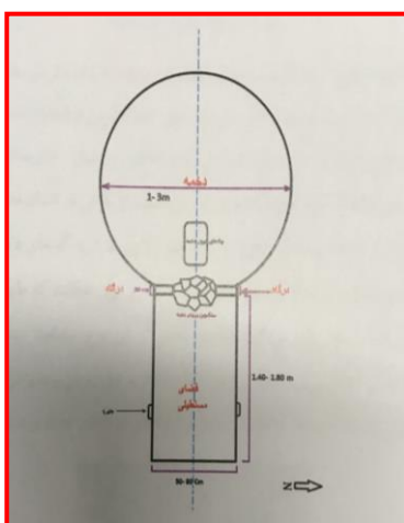
تصویر-۸: پلان گور دخمه ها دوره اشکانی، گورستان وستمین (شریفی: ۱۳۹۵، ۲۴۷-۲۴۶)
