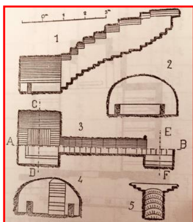
طرح و پلان ۲- قبور چاهی آکروپل و شهر شاهی در شوش (سعیدی: ۱۳۷۵، ۲۱۷) پلان و مقطع ۳- آرامگاه سردابه ای پارتی در شهر صنعتگران شوش (چاپچی و سعیدی: ۱۳۸۱، ۱۲۷)
