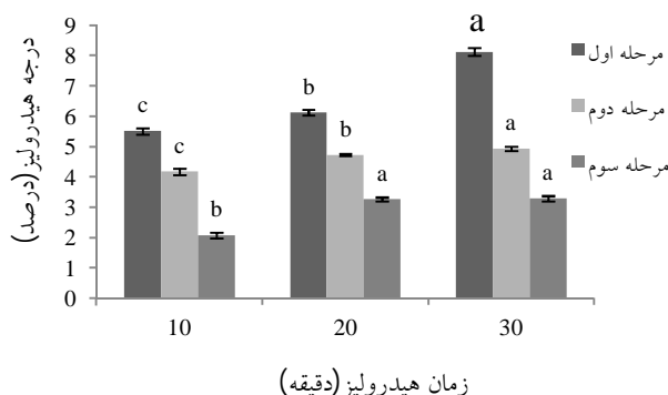
شکل 4- تأثیر زمان بر درجه هیدرولیز در مراحل اول، دوم و سوم هیدرولیز
