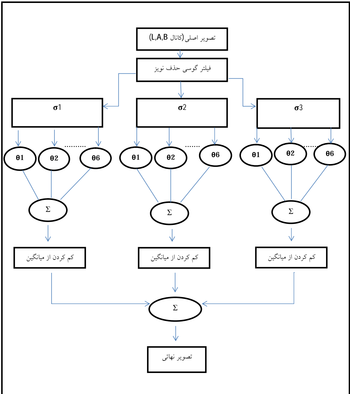
شکل 1 - الگوریتم پیشنهادی
