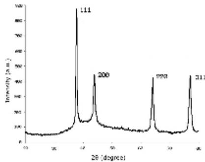
شکل 3- الگوی XRD نانوذرات نقره
