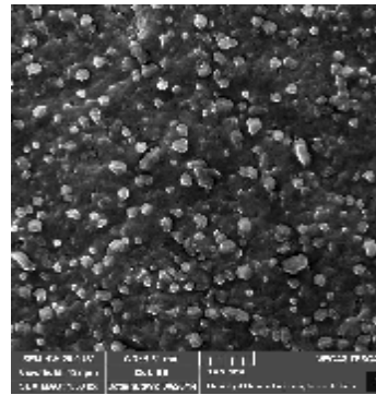
شکل 4- تصاویر SEM از نانوذرات نقره تشکیل شده به وسیله تبدیل از نیترات نقره 1 میلی مولار و عصاره آبی بذر بادیان رومی
