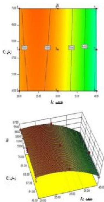
شکل 5- تاثیر زمان و غلظت خاک بنتونیت بر رنگ ملاس
