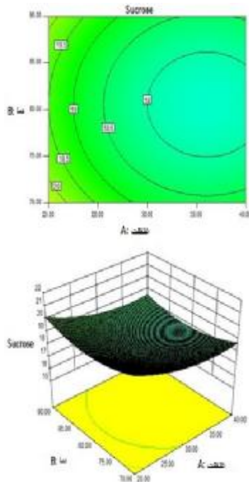
شکل 3- تاثیر دما و غلظت خاک بنتونیت بر ساکارز ملاس
