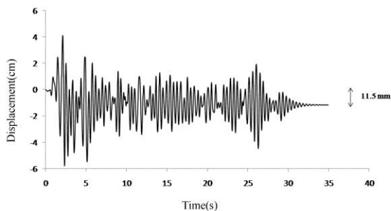
شکل ۵- تاریخچه زمانی تغییر مکان افقی تراز طبقه سوم در سیستم مهاربند فولادی مقاوم در برابر کمناش بدست آمده از تحلیل ANSYS
