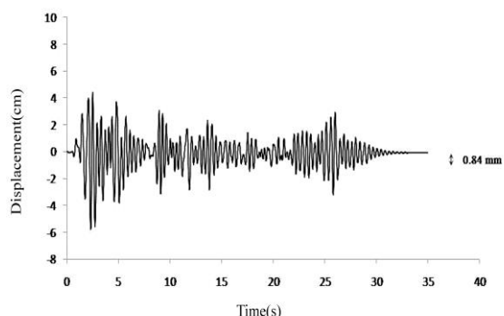
شکل ۱۸- تاریخچه زمانی تغییرمکان افقی تراز طبقه سوم در سیستم مهاربندی با ترکیب SMA 100% و Steel 0% تحت حداکثر شتاب 0.6g
