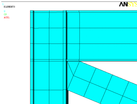
شکل ۱۴- نحوه مش بندی و اتصال مهاربند به تیر- ستون
