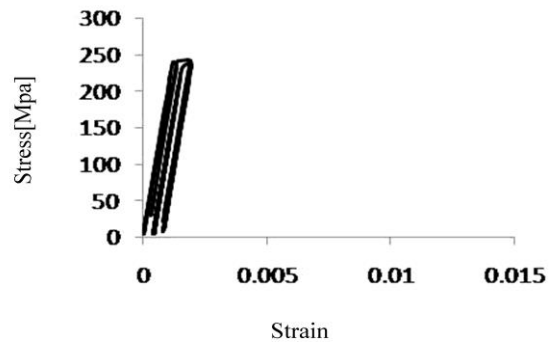
شکل ۲۲- نمودار هیستریزیس مهاربند SMA (مدل ششم) تحت حداکثر شتاب 0.9g
