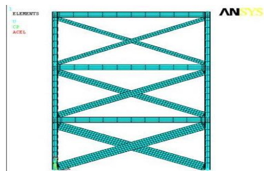
شکل ۱۳- نحوه مدل سازی قاب در ANSYS
