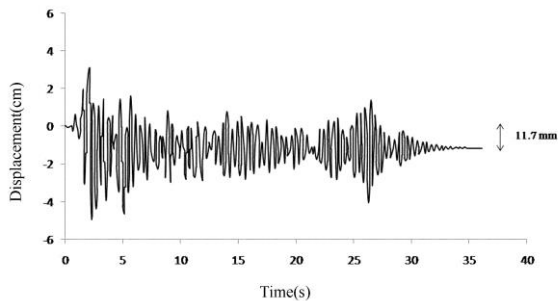
شکل ۴- تاریخچه زمانی تغییر مکان افقی تراز طبقه سوم در سیستم مهاربند فولادی مقاوم در برابر کمناش بدست آمده از نتایج کاری [۲۱]
