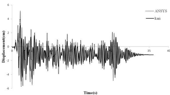
شکل ۶- مقایسه تاریخچه زمانی تغییر مکان افقی تراز طبقه سوم در سیستم مهاربند فولادی مقاوم در برابر کمناش بدست آمده از تحلیل ANSYS و نتایج کاری
