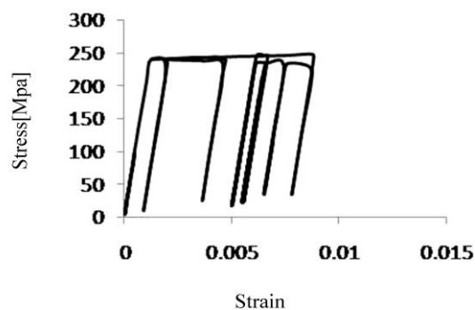
شکل ۲۶- نمودار هیستریزیس مهاربند فولادی (مدل اول) تحت حداکثر شتاب 0.9g
