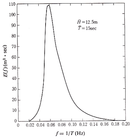
شکل ۳- طیف برتشنايدر
