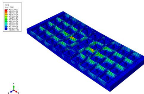
شکل ۶- کرنش های ایجاد شده در مقطعی از دال یوبوت
