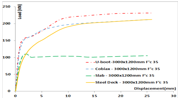
شکل ۱۳- مقایسه منحنی نیرو-جابجایی سقف یوبوت با نمونه‌های دال بتنی-کوبیاسکس و عرشه فولادی مرجع دارای بتن با مقاومت ۳۵ مگاپاسکال [۱۱]
