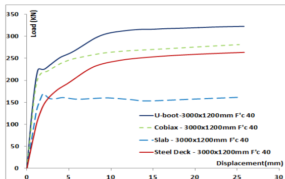
شکل ۱۴- مقایسه منحنی نیرو-جابجایی سقف یوبوت با نمونه‌های دال بتنی-کوبیاسکس و عرشه فولادی مرجع دارای بتن با مقاومت ۴۰ مگاپاسکال [۱۱]
