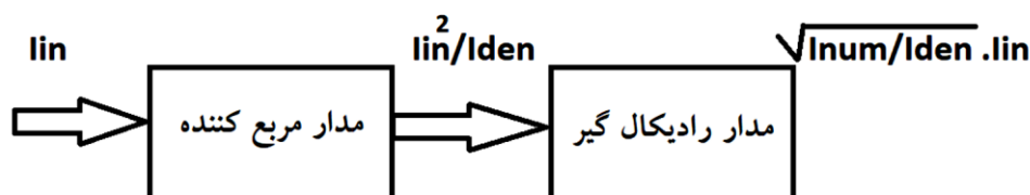
شکل ۱۸: نحوه‌ی تولید مدار ضرب کننده برای ایجاد یک ضریب برای تنظیم شیب و یا ضرایب تقریب توان
