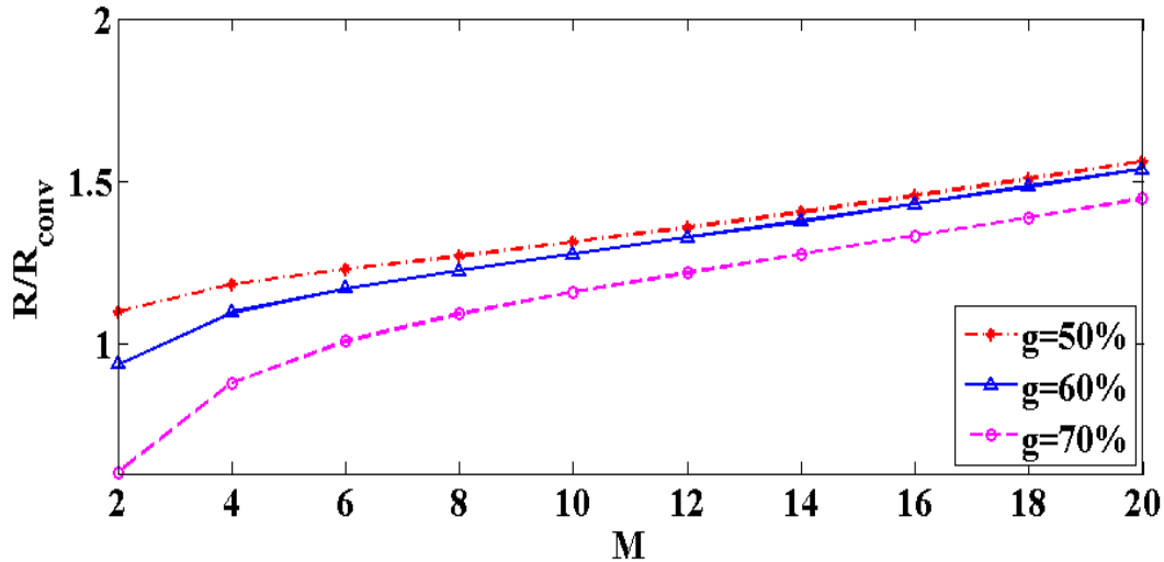
شکل ۶: کارایی گذردهی به عنوان تابعی از تعداد کاربران ثانویه (SNR=-16dB) Figure 6. Throughput efficiency as a function of the number of secondary users (SNR=-16dB)
