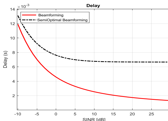
شکل (۹): مقایسه تاخیر با افزایش مقدار SINR در شبکه پیشنهادی و روش شکل دهنده پرتو هماهنگ
