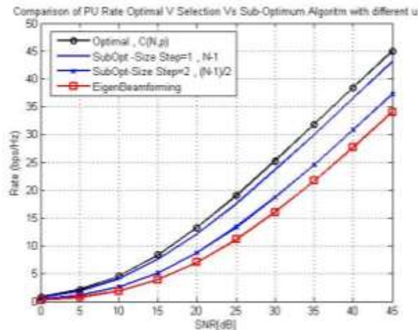
شکل (۴): نرخ کاربر اولیه در استراتژی افزایش نرخ اولیه برای مقایسه عملکرد روش گزینش بردار پرتودهی کارآمد و زیر بهینه با دو اندازه گام u=2 و u=1 و روش همسونهی تداخل پرتودهی ویژه
