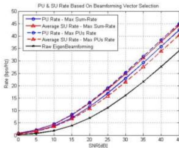
شکل (۲): مقایسه دو استراتژی نرخ شبکه با استفاده از روش گزینش بردار پرتودهی کارآمد
