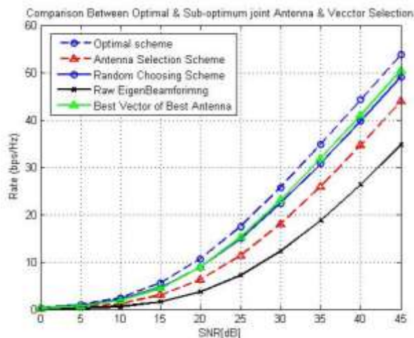
شکل (۷): نرخ کاربر اولیه در استراتژی افزایش نرخ کاربر اولیه با استفاده از روش‌های کارآمد، روش گزینش تصادفی، گزینش بهترین بردار بهترین آنتن و همچنین طرح همسونهی تداخل پرتو دهی ویژه
