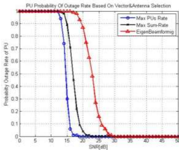
شکل (۶): احتمال نرخ انقطاع کاربر اولیه با توجه به دو استراتژی نرخ شبکه با استفاده از روش گزینش بردار پرتودهی و آنتن تواما
