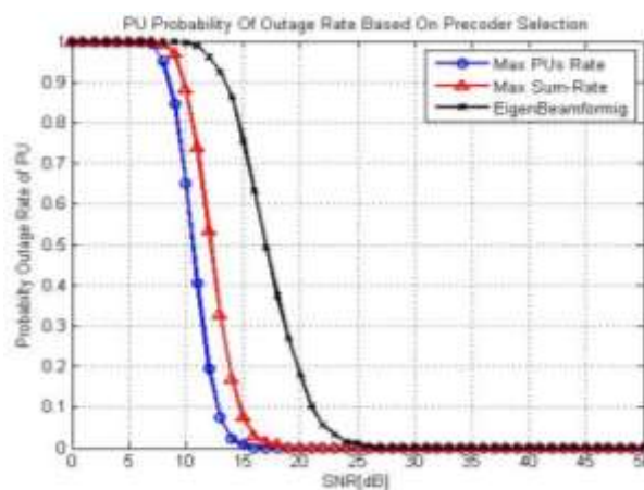
شکل (۳): احتمال نرخ انقطاع کاربر اولیه با توجه به دو استراتژی نرخ شبکه با استفاده از روش گزینش بردار پرتودهی
