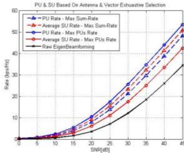
شکل (۵): مقایسه دو استراتژی نرخ شبکه با استفاده از روش گزینش بردار پرتودهی و آنتن تواما
