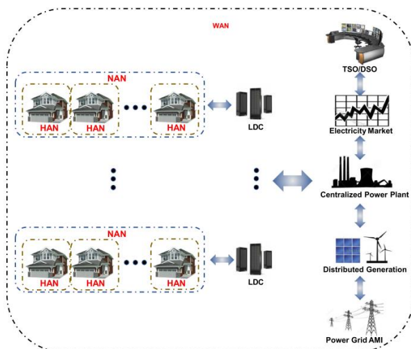
شکل (۹): زیرساخت ارتباطی شبکه هوشمند برق [۴۰]
