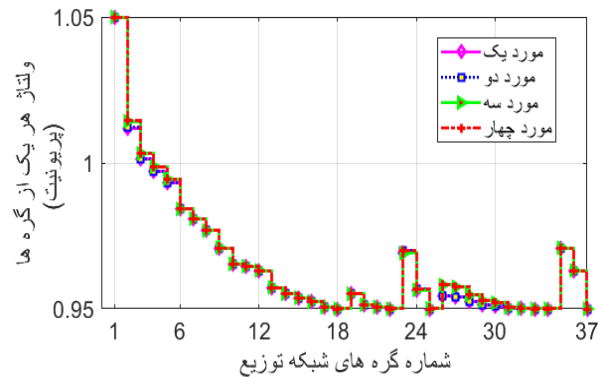
شکل (۸): پروفیل ولتاژ هر یک از گره‌های شبکه (پریونیت)
