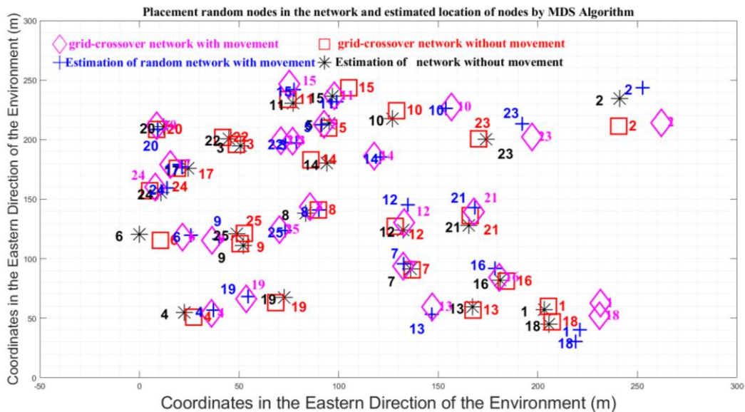
شکل (۱۲): قرارگیری گره‌های تصادفی در مکان تخمین زده‌شده‌ی گره‌ها توسط روش MDS
