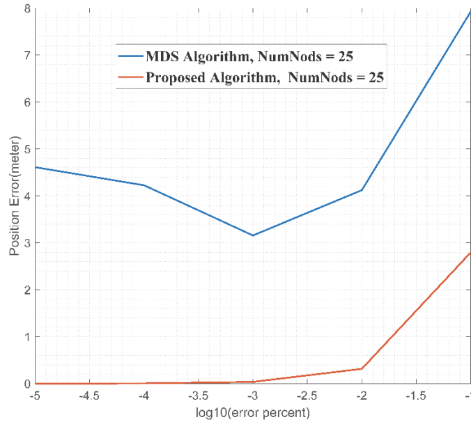
شکل (۱۱): منحنی‌های خطای مکان‌یابی شبکه‌ی گرید- متقاطع
