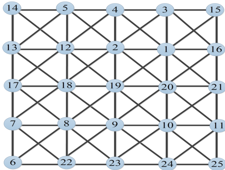
شکل (۵): مکان گره‌های شبکه‌ی گرید با اتصال متقاطع Figure (9): the location of nodes of the grid network with cross-connection
