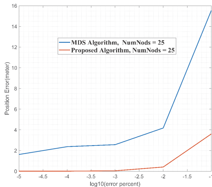
شکل (۸): منحنی‌های خطای مکان‌یابی شبکه‌ی گرید متقاطع Figure (8): Grid – crossover location positioning error curves
