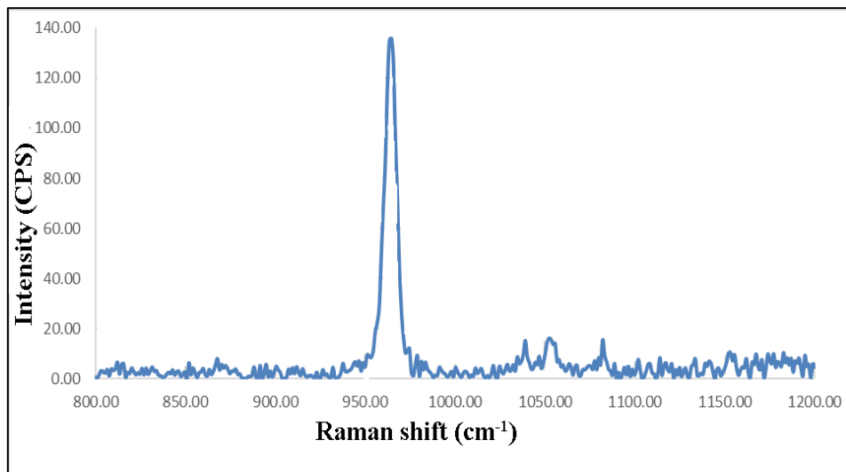
Fig. 11. Flourapatite spectroscopy test
