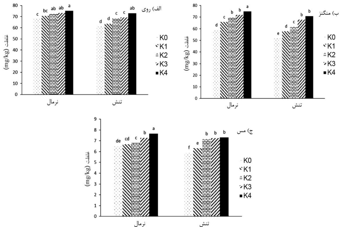
شکل ۱: مقایسه میانگین اثر متقابل پتاسیم و تنش خشکی بر غلظت عناصر غذایی کم مصرف (الف-روی، ب-منگنز و ج-مس) در برگ لوبیا چشم بلبلی. K0- k4 به ترتیب مقادیر پتاسیم (صفر، ۳۰، ۶۰، ۹۰ و ۱۲۰ میلی‌گرم برکیلوگرم) می‌باشند. میانگین‌های دارای حروف مشترک بر اساس آزمون دانکن در سطح احتمال ۵ درصد با همدیگر اختلاف معنی‌داری ندارند.
