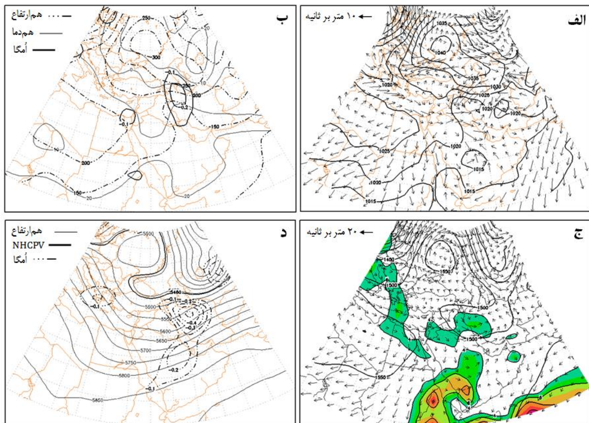
شکل ۱۰: نقشه‌های ۲۴ ژانویه ۲۰۰۱؛ (الف) هم فشار سطح دریا و سرعت باد؛ (ب) هم ارتفاع، هم دما و اُمگا در تراز زمین؛ (ج) هم ارتفاع، جریان باد و نم ویژه در تراز 850 \text{ hp} ؛ (د) هم ارتفاع، تاوه پیراقطبی و اُمگا در تراز 500 \text{ hp} .
