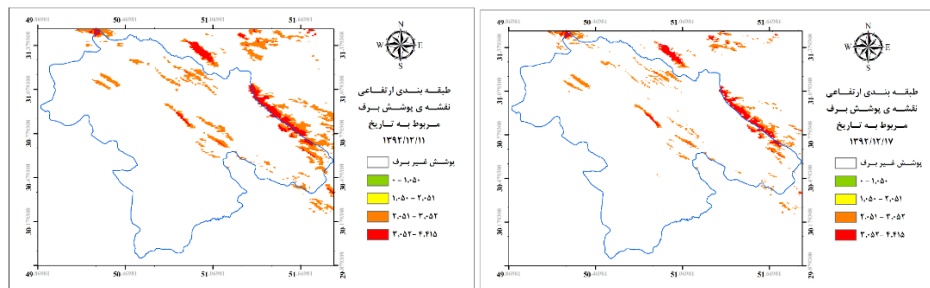
شکل (۶): تلفیق نقشه برف عاری از ابر و مدل رقومی شده
