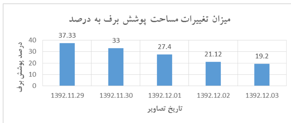
شکل (۳): مقدار پوشش برف تصاویر ماهواره‌ای
