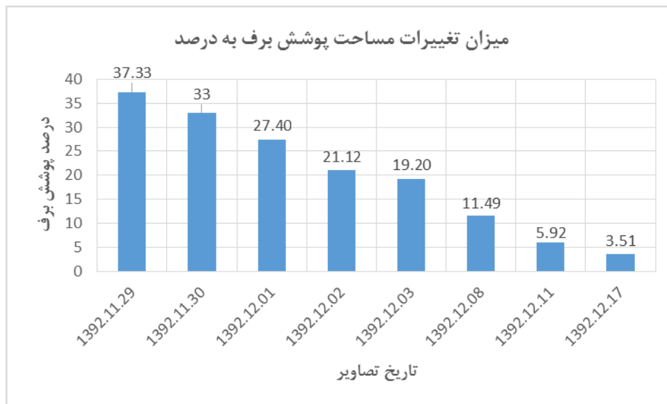
شکل (۵): مقدار پوشش برف تصاویر ماهواره‌ای در بازه‌ی زمانی مورد بررسی و در سه تاریخ ۹۲/۱۲/۱۷ و ۹۲/۱۲/۱۱، ۹۲/۱۲/۰۸
