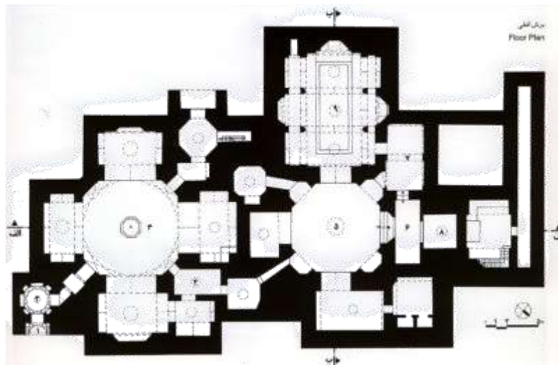
۱. تصویر ۱. پلان حمام ایرانی (حمام شاه اصفهان)؛ مأخذ: گنج‌نامه. ۱. ورودی ۲. هشتی ۳. بینه ۴. میان‌در ۵. گرم‌خانه ۶. خزینه ۷. شاه‌نشین ۸. تیان ۹. چال‌حوض.
