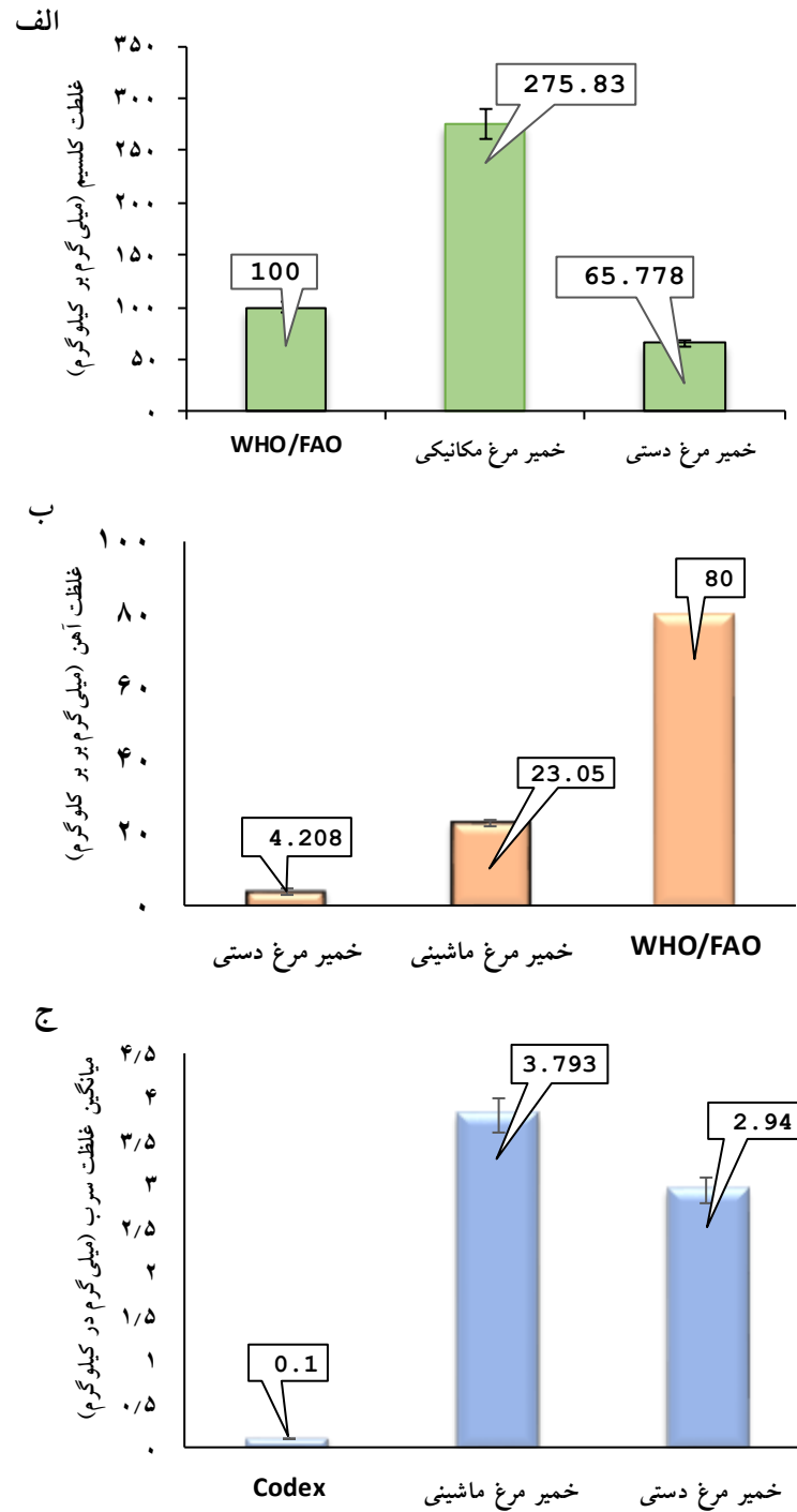
نمودار (۱) - مقایسه میانگین غلظت کلسیم (الف)، آهن (ب) و سرب (ج) در نمونه‌های خمیر مرغ (روش دستی و مکانیکی) با حدود مجاز اعلام‌شده از سوی استانداردهای بین‌المللی
