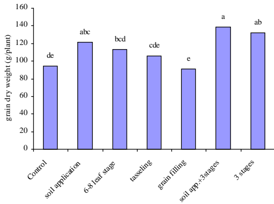
شکل ۷- اثر نحوه و زمان مصرف روی بر عملکرد خشک دانه Figure 7- Effect of method and time of Zn application on yield of dry grain
