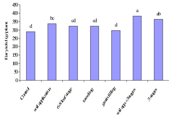
شکل ۶- اثر نحوه و زمان مصرف روی بر عملکرد بلال ذرت شیرین
