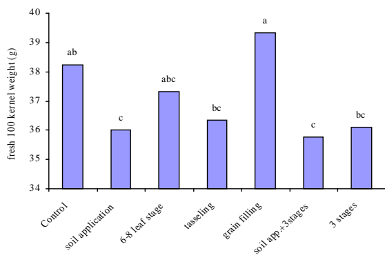
شکل ۵- اثر نحوه و زمان مصرف روی بر وزن صد دانه تر
