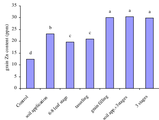
شکل ۱۱- اثر نحوه و زمان مصرف روی بر تعداد بلال ذرت شیرین Figure 11- Effect of method and time of Zn application on grain Zn content
