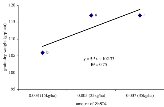
شکل ۹- اثر میزان مصرف روی بر تعداد بلال ذرت شیرین Figure 9- Effect of Zn amount uses on yield of dry grain
