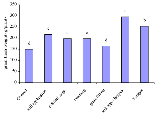
شکل ۸- اثر نحوه و زمان مصرف روی بر عملکرد تر دانه Figure 8- Effect of method and time of Zn application on yield of fresh grain
