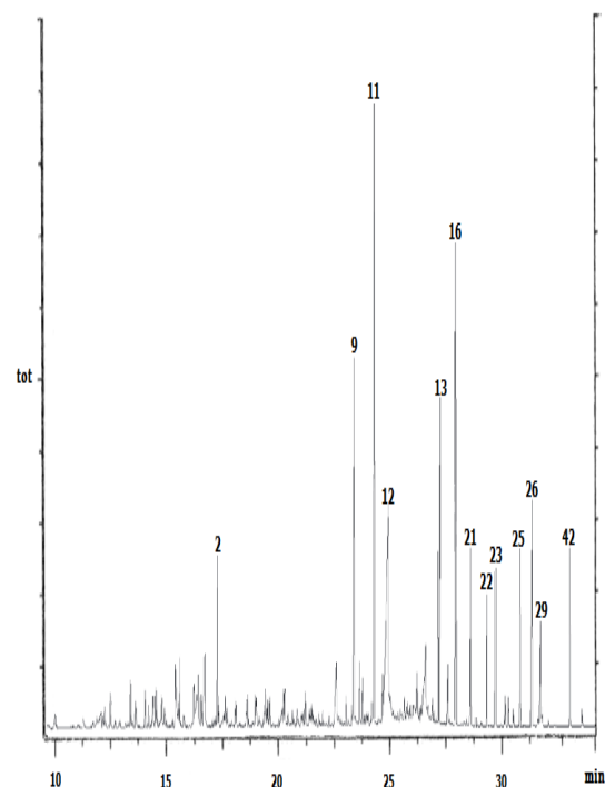
شکل ۱: کروماتوگرام GC اسانس گیاه دارویی زنجبیل (Zingiber officinale)
