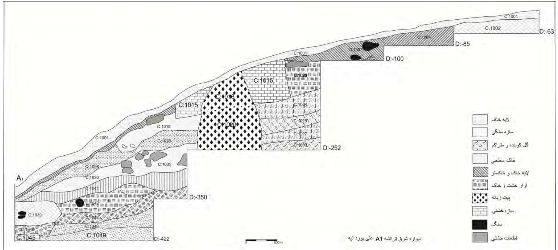
تصویر ۳: طرح برش دیواره شرقی ترائشه A1.
