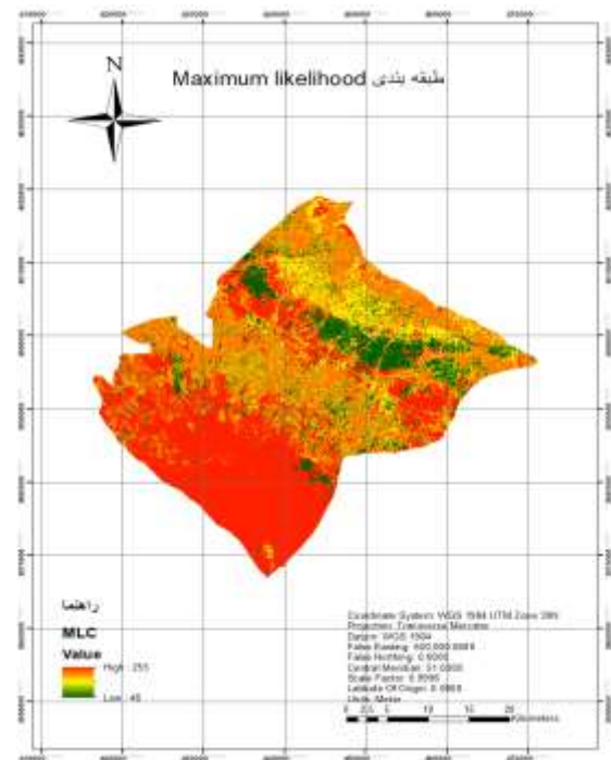
شکل (۳). طبقه بندی به روش MLC
