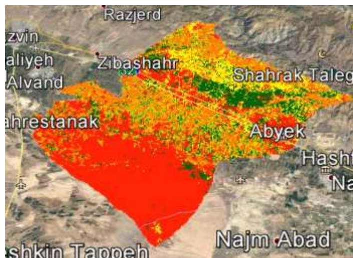
شکل (۶). نقشه الگوریتم MLC در Google Earth (محدوده آبیک)، منبع: نگارندگان، ۱۳۹۹
