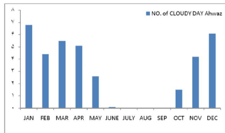
شکل ۴ میانگین ماهانه تعداد روزهای با آسمان ابری
