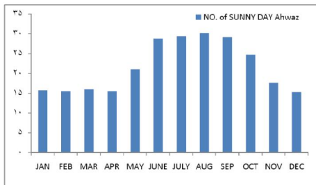
شکل ۳ میانگین ماهانه تعداد روزهای با آسمان آفتابی
