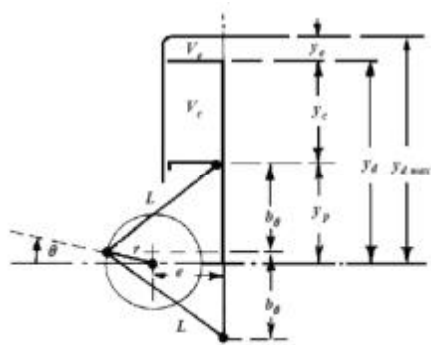
شکل 3 مکانیزم عملکرد و تغییرات حجم در موتور استرلینگ نوع بتا
