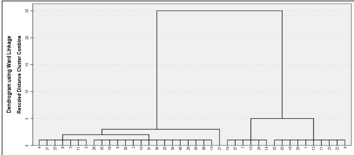
شکل ۵- نمودار خوشه ای برای نمونه های آب زیرزمینی منطقه
