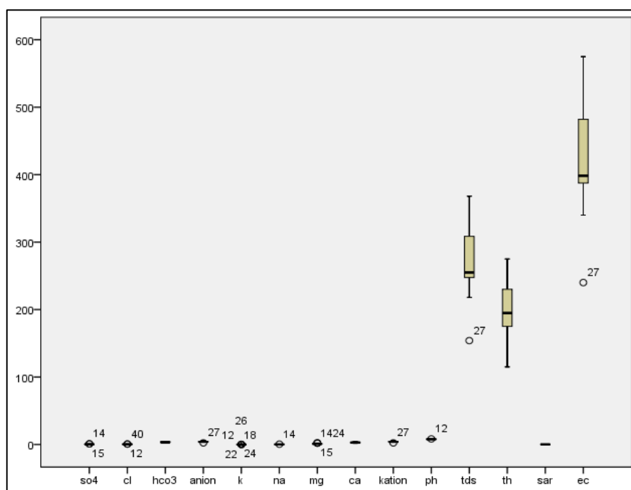
شکل ۴- نمودار جعبه ای متغیرهای فیزیکوشیمیایی آب زیرزمینی منطقه
