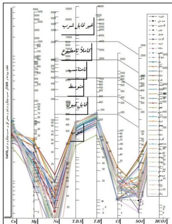
شکل ۸- نمودار شولر برای نمونه های آب زیرزمین
