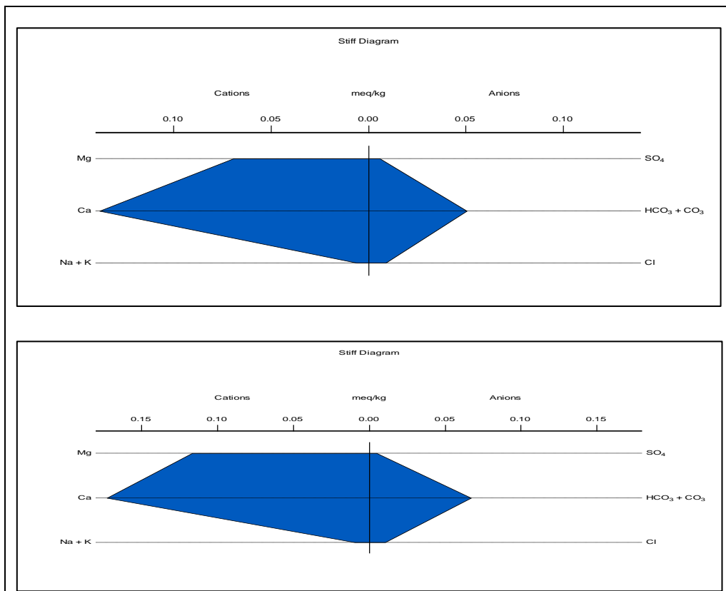
شکل ۶- نمودار استیف مربوط به خوشه یک (بالا) و خوشه دو (پایین)
