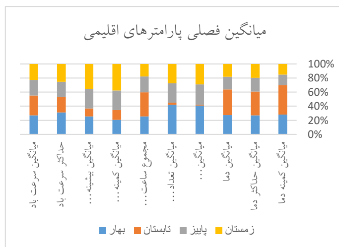
شکل ۳: پارامترهای اقلیمی سبزواری طی دوره آماری ۱۳۹۴ تا ۱۳۹۹.
