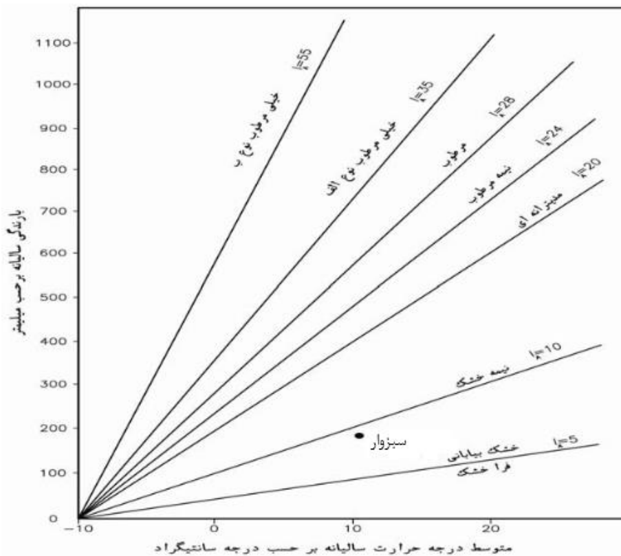
شکل ۲: موقعیت اقلیمی شهرستان سبزوار در اقلیم نمای دومارتن
