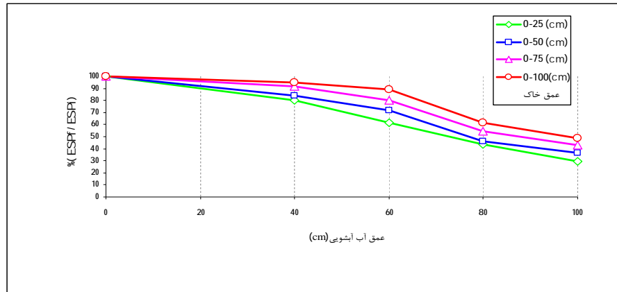
شکل 2: رابطه بین میزان آب آیشویی و درصد سدیم تبدالی در لایه‌های مختلف نیمرخ خاک
