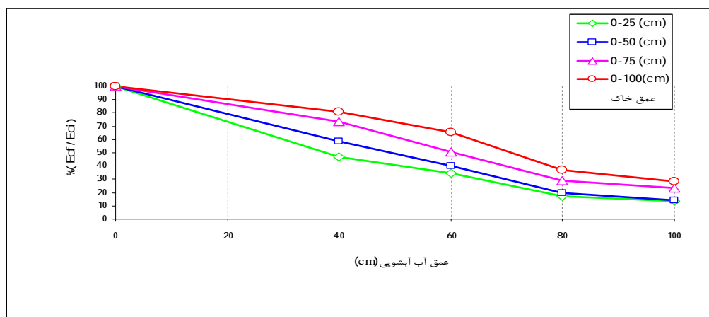
شکل 1: رابطه بین میزان آب آبشویی و درصد شوری در لایه های مختلف نیمرخ خاک
