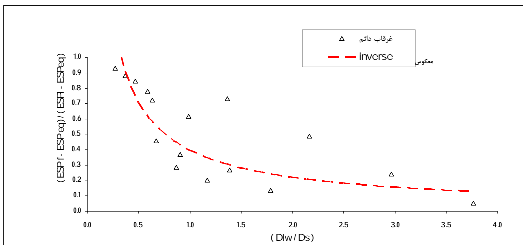
شکل 4: منحنی سدیم زدایی
