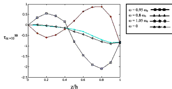
نمودار (۳): تغییرات تنش \sigma_z ، \tau_{rz} با \omega های مختلف در ضخامت های مختلف از ورق
