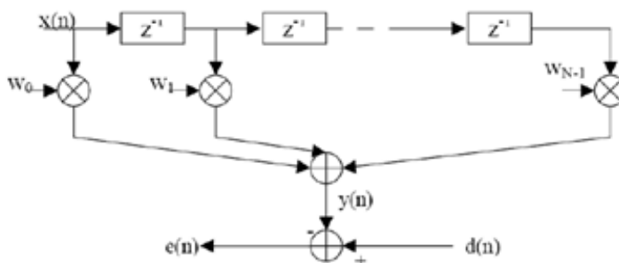
فرایند الگوریتم LMS و فیلترینگ عرضی
