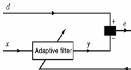
شکل ( 1 ) : ساختار کلی فیلتر وفقی
