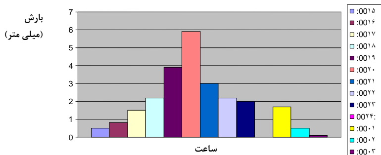
شکل ۵- مقدار بارش کل در تاریخ 11.10.2006
