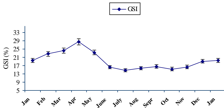
نمودار ۱- روند تغییرات مقدار میانگین شاخص گنادی (GSI) در ماهی سفید دریای خزر به تفکیک ماه. Diagram 1- Average gonado-somatic index (GSI) fluctuation of Caspian Sea Kutum (monthly).
