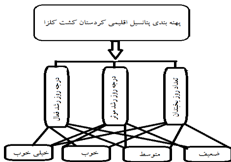
شکل ۲- ساختار سلسله مراتبی پهنه‌بندی کشت کلزا Figure 2. Analytic hierarchy process for canola cultivation regionalization
