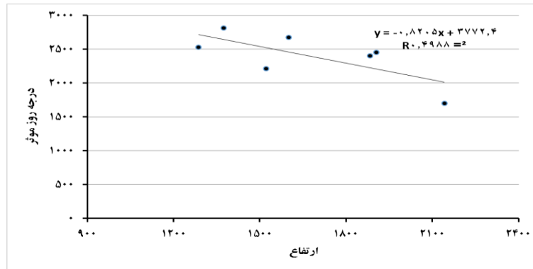
شکل ۸- همبستگی درجه روز موثر گیاه کلزا با ارتفاع
