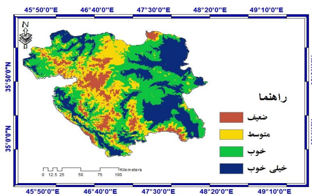
شکل ۱۳- پهنه‌بندی تناسب اراضی استان کردستان جهت کشت کلزا با مدل فازی و AHP
