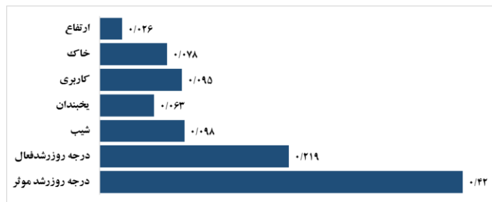
شکل ۳- وزن و ضریب اهمیت هر لایه اقلیمی در پهنه‌بندی کشت کلزا در کردستان
