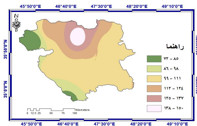
شکل ۱۰- طبقه‌بندی تعداد روز یخبندان در استان کردستان
