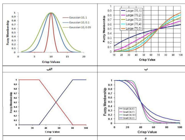
شکل ۴- توابعی که برای فازی سازی معیارها استفاده شده است (الف). تابع گوسی (زنگوله ای) (ب: تابع large (ج). تابع خطی s شکل. (د). تابع small
