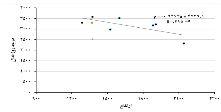
شکل ۶- همبستگی درجه روز فعال گیاه کلزا با ارتفاع
