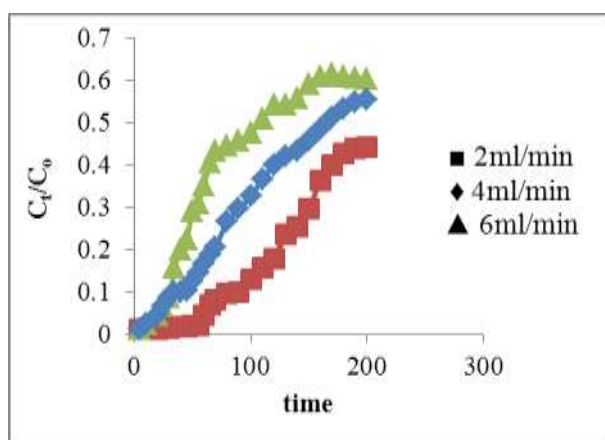
شکل ۹- منحنی شکست برای حذف مس در بستر جاذب تثبیت شده در سرعت جریان های مختلف ( C_0=5\text{ppm} ) pH=5/5، ارتفاع بستر = 20cm
