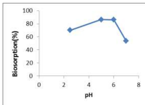
شکل ۴- اثر تغییرات pH در جذب سطحی Cu(II) به وسیله جاذب در شرایط (۱۰۰ml محلول ۵ppm از مس، دمای محلول، سرعت ۱۵۰rpm، ۱g قارچ)
