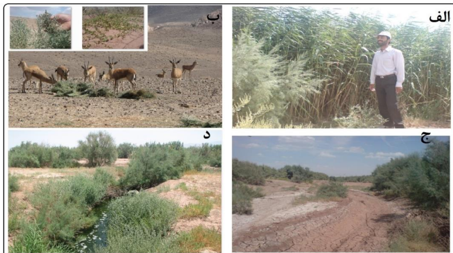
شکل ۷- (الف) نی‌زارهای بستر رودخانه کال شور (ب). نمونه‌ای حیات جانوری و گیاهی منطقه حفاظت شده شیر احمد (ج) بستر رودخانه کال شور در فصل کم آبی (د) ورود پساب تصفیه شده به اکوسیستم آن و تاثیرات منفی آن منطقه Figure 7. (A) Flaggy in river bed of kalshour (B) An example of animal and plant life in a protected area ShirAhmad (C) Kalshour river bed during the dry season (D) Wastewater entering the river ecosystem and its negative impact area
