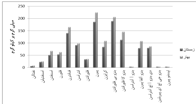
نمودار ۱- مقایسه میانگین ترکیبات PAHs در دو فصل زمستان و بهار
