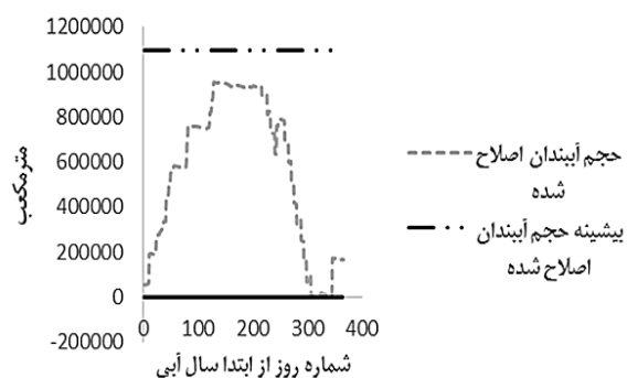
شکل ۶. تغییرات حجم آب ذخیره شده در آب‌بندان اصلاح شده در سال آبی مورد بررسی
