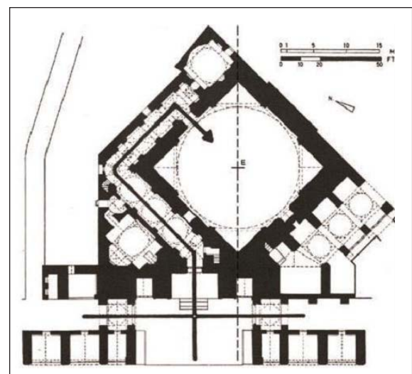
شکل ۲. پلان مسجد شیخ لطف الله (ماخذ: پیرنیا، ۱۳۸۳)
